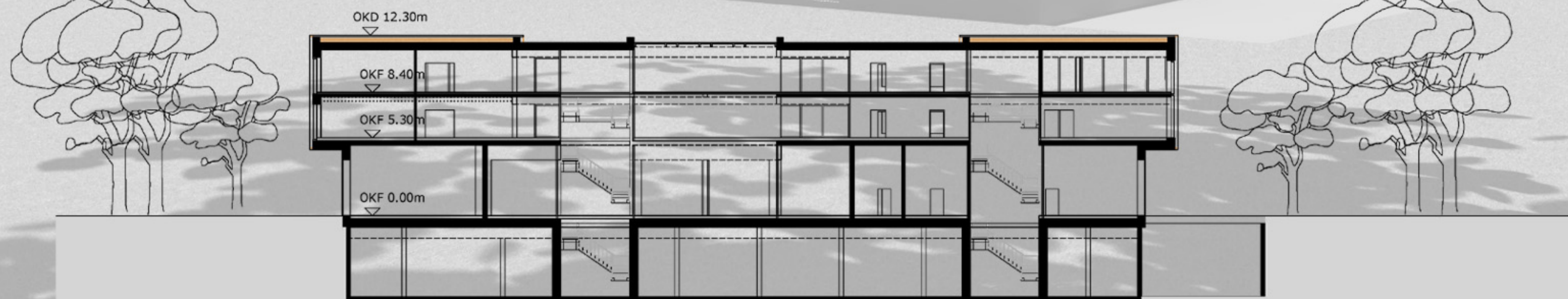
Schnitt DD
